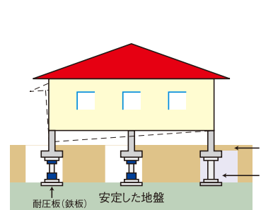
耐圧板工法
