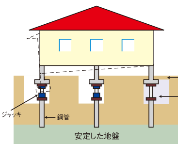
鋼管杭圧入工法 (アンダーピーニング工法)
